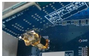
Рисунок 6.4 — GSM-антенна STEMAX AMG02, установленная на плате контроллера
