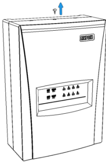
Рисунок 6.1 — Демонтаж корпуса контроллера (шаг 1)
