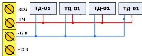
Рисунок 6.6 — Схема подключения цифровых датчиков температуры Мираж-ТД-01
