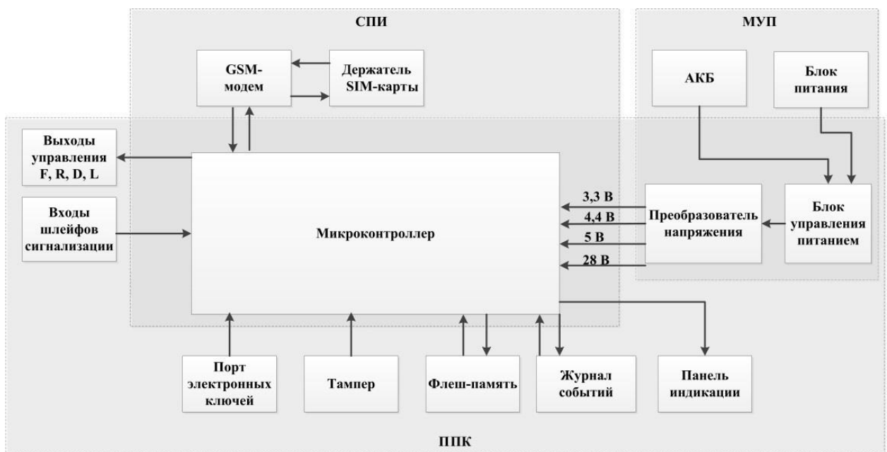
Рисунок 5.1 — Функциональная схема
