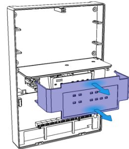
Рисунок 6.3 — Демонтаж корпуса контроллера (шаг 3)
