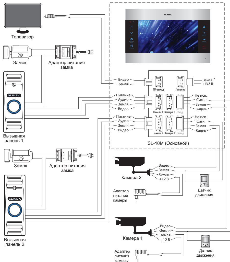
Схема 1. Подключение вызывных панелей, камер и телевизора к домофону SL-10M.
