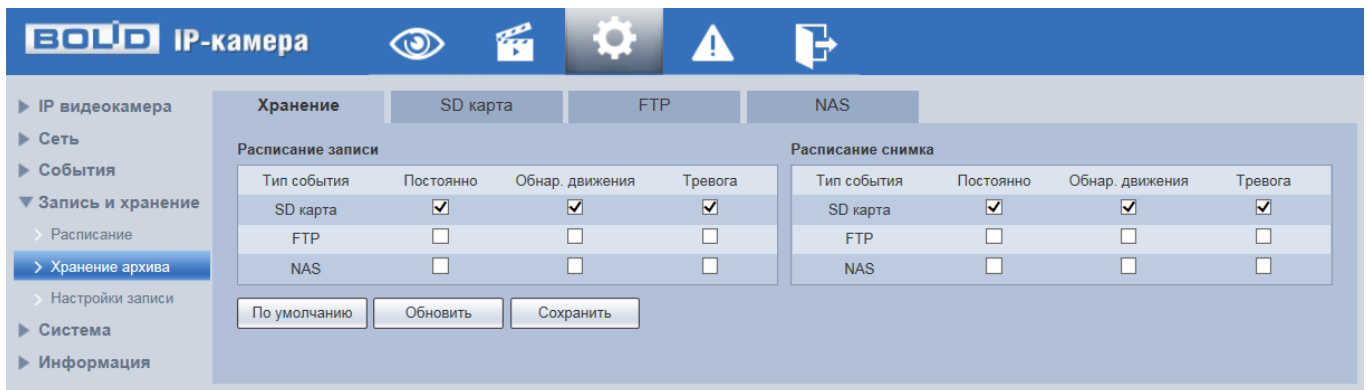
Рисунок 7.100 – Вкладка «Хранение»
