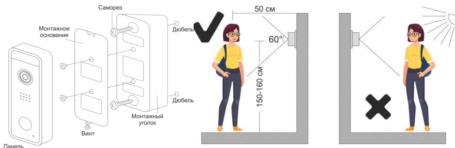
Рисунок 4. Схема установки панели
