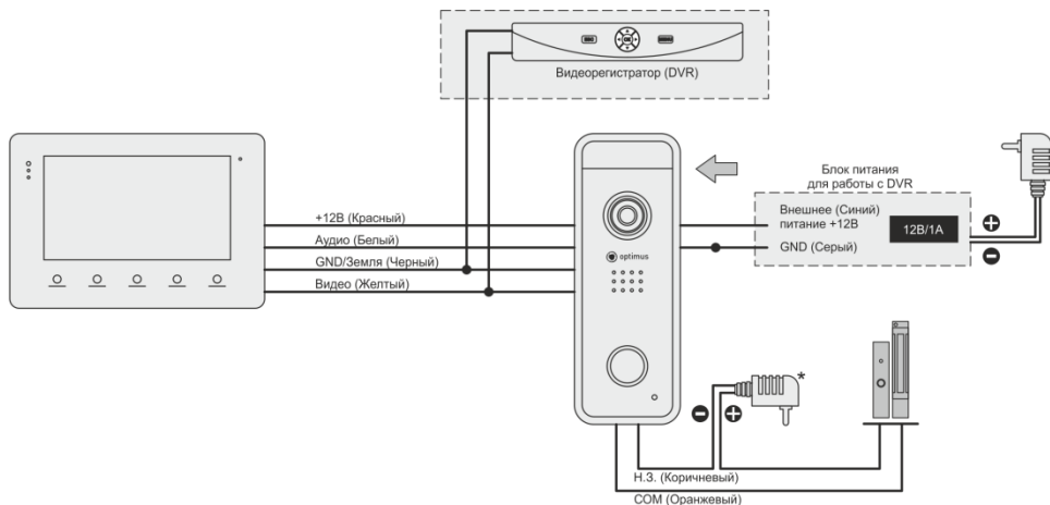
Рисунок 3. Схема подключения №3
