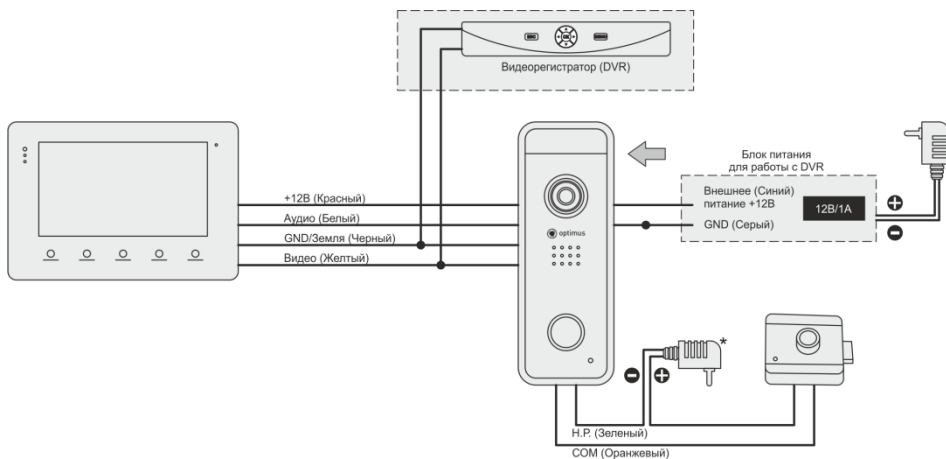
Рисунок 2. Схема подключения №2
