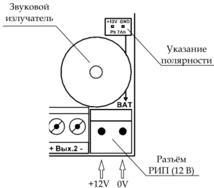
Рисунок 2.2.6 Схема подключения РИП 12 В
