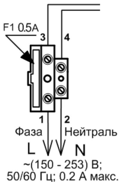
Рисунок 2.2.5 Схема подключения ОИП 230 В
