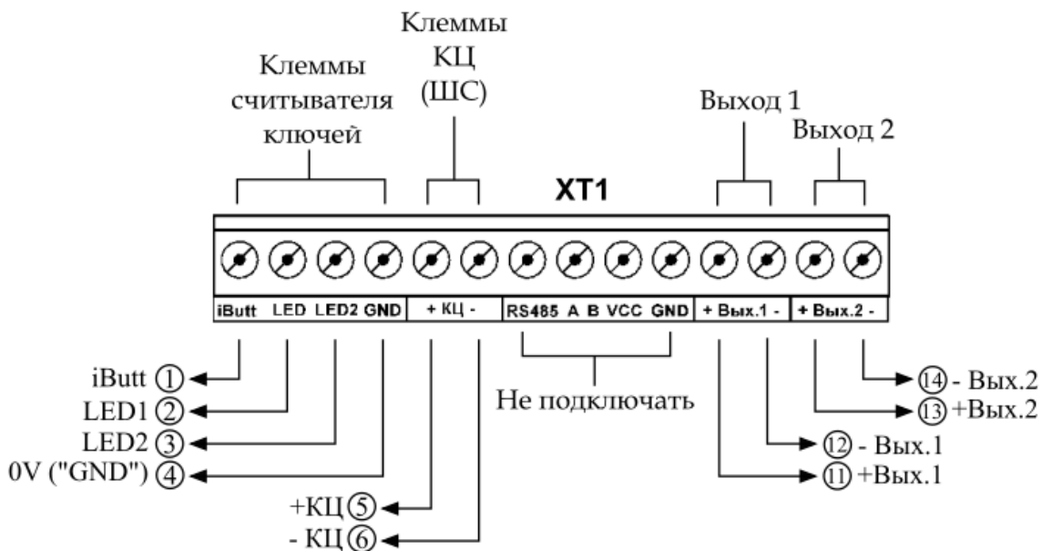
Рисунок 2.2.7 Схема внешних подключений
