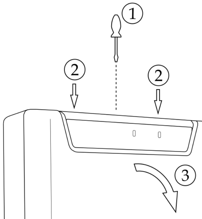
Рисунок 2.2.2 Вскрытие корпуса
