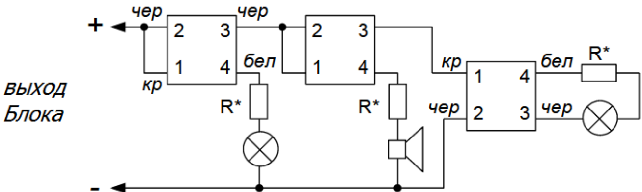
Рисунок 2.2.4.4.3 Схема подключения нескольких оповещателей устройств ( R^* - токоограничивающие резисторы, исходя из максимального тока нагрузки выхода)
