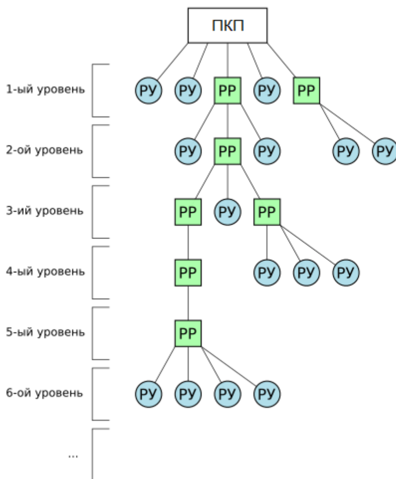
Рисунок 1.4.1 Цепь ретрансляции
