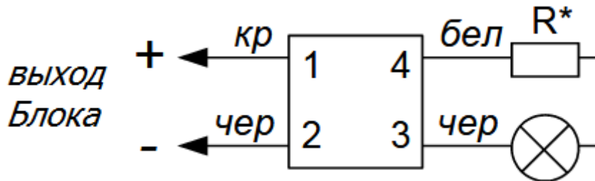
Рисунок 2.2.4.4.2 Схема подключения одиночного оповещателя ( R^* – токоограничивающий резистор, исходя из максимального тока нагрузки выхода)
