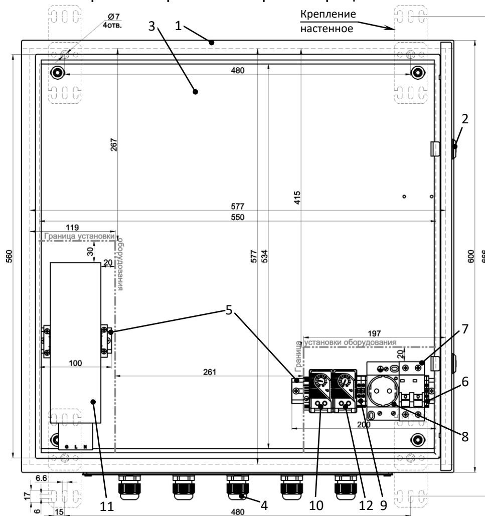
Рисунок 1 – Устройство шкафа
